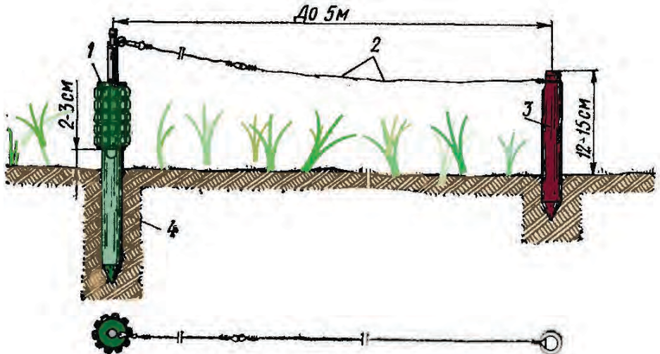
Малюнок 6.2.2 – Міна ПОМЗ-2М, встановлена на ґрунті: 1 – міна; 2 – дрова розтяжка; 3,4 – дерев'яний кілок. На нижньому малюнку – вигляд зверху
