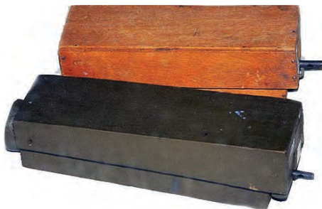
Міна ПМД-6М, маркування та забарвлення
