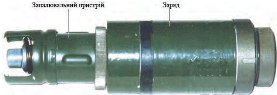
Малюнок 12.1.1 – Міна-граната ЗМГ, загальний вигляд
