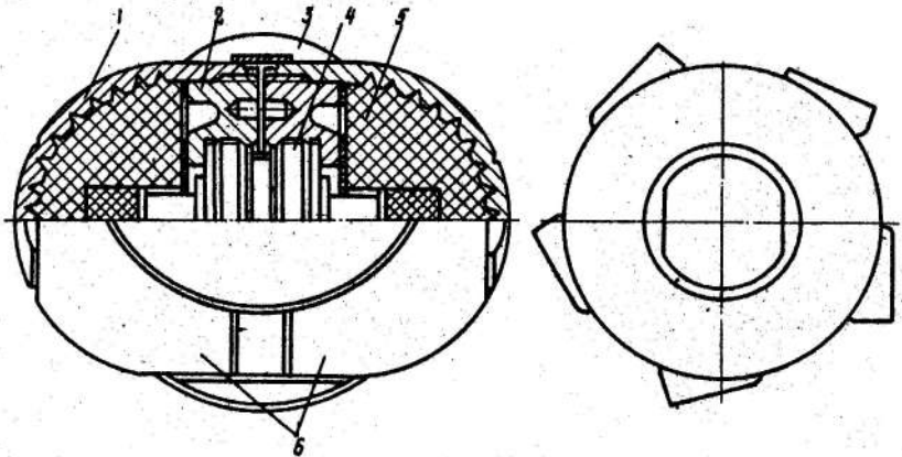
РИС. 8. АВИАБОМБА АО-2,5РТ:
