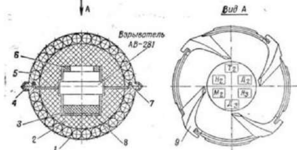
Рис. 6. Шариковая осколочная авиабомба ШОАБ-0,5:
