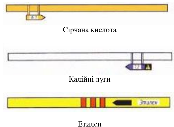
Рисунок 3.2 – Приклади маркування трубопроводів промислових підприємств
