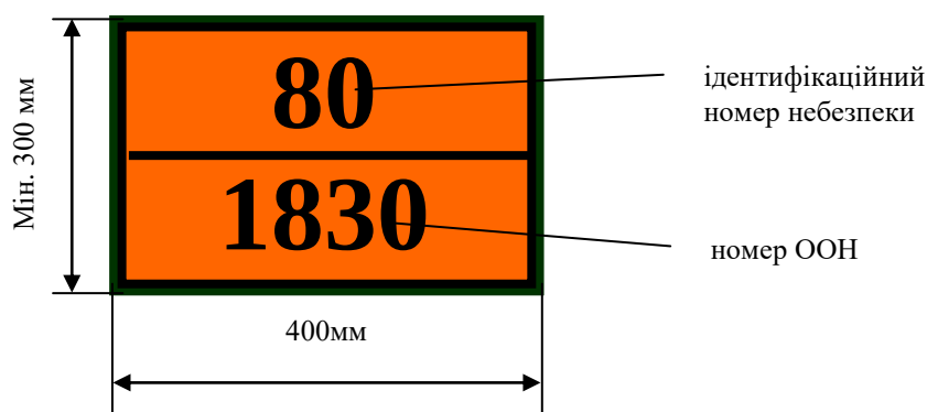
Рисунок 3.5 – Приклад інформаційної таблички оранжевого кольору з ідентифікаційним номером небезпеки та номером ООН
